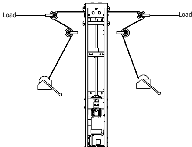
Proporcion 2:1 (Figura 11)
