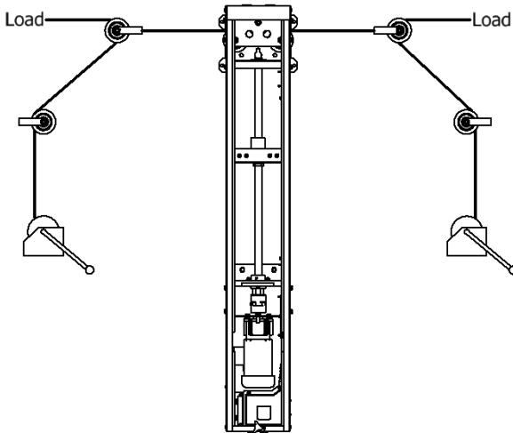
Proporcion 2:1 (Figura 11)
