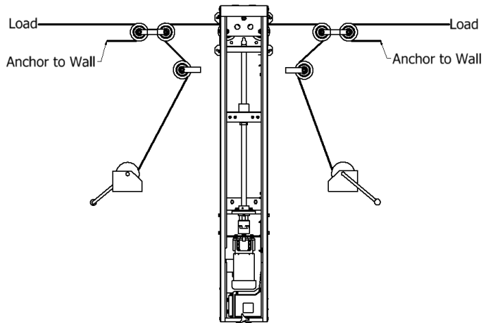
Proporcion 1:1 (Figura 9)
