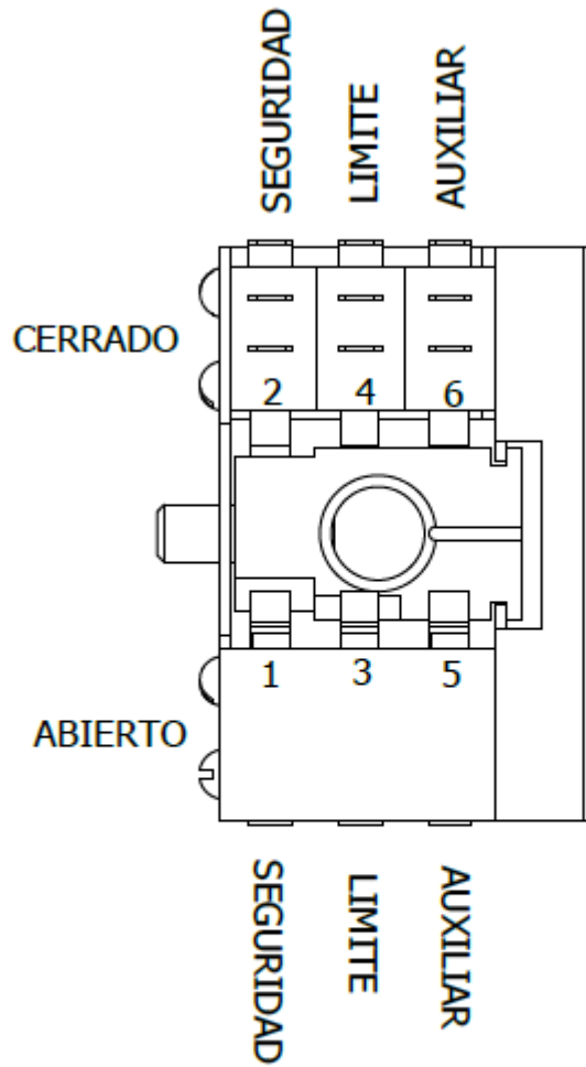
VISTA SUPERIOR DE ENSAMBLE DE INTERRUPTOR
